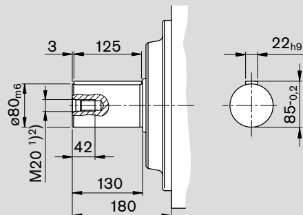
P Clavette DIN 6885 AS22x14x125
