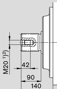
Z Arbre cannelé DIN 5480 W80x3x25x9g
